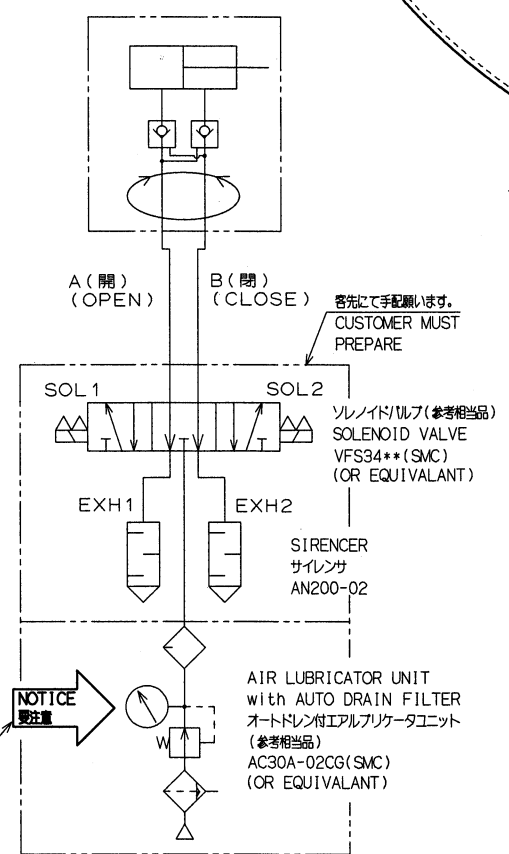
エア回路図 AIR DIAGRAM
