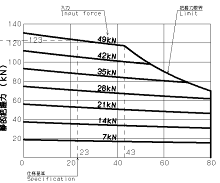
把握部中心高さ (mm) Gripping center height
