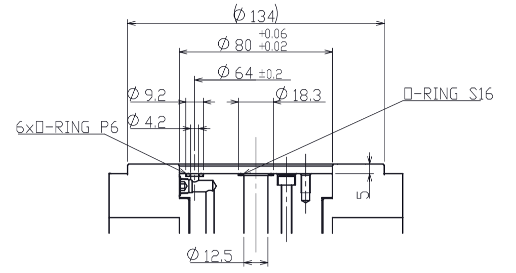
テーブル面詳細 DETAIL OF TABLE (1:2)
