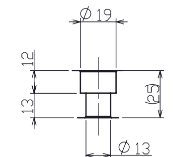
クランプ部詳細(10か所) DETAIL OF CLAMP HOLE (10 PLACES) (1 : 2)
