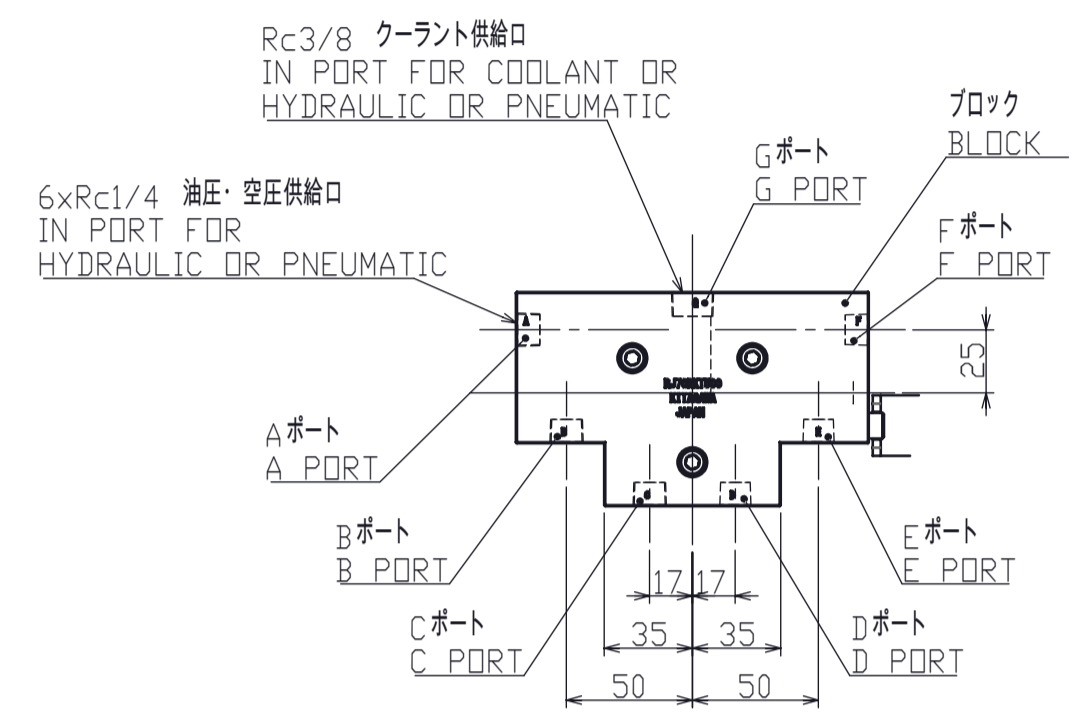
シグ用配管接続位置詳細 (1 : 3)
